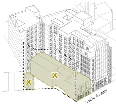
01 - Demolição de galpão existente não tombado
